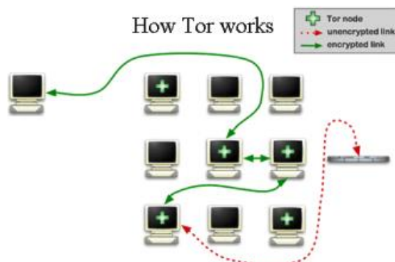
Slika 2: Način rutiranja internet paketa u Tor mreži. [21]
